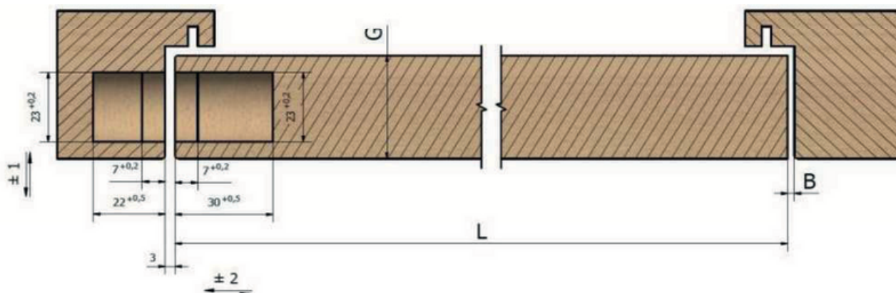
Posición de la visagra en relación con las dimensiones requeridas de la puerta y del marco
